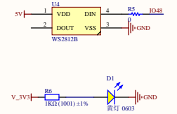
指示灯
