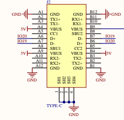
标准USB接口
