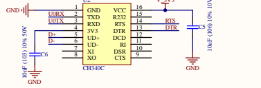
串口烧录电路
