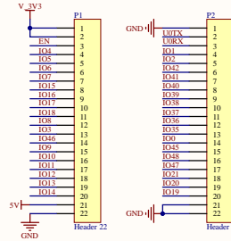
扩展引脚
